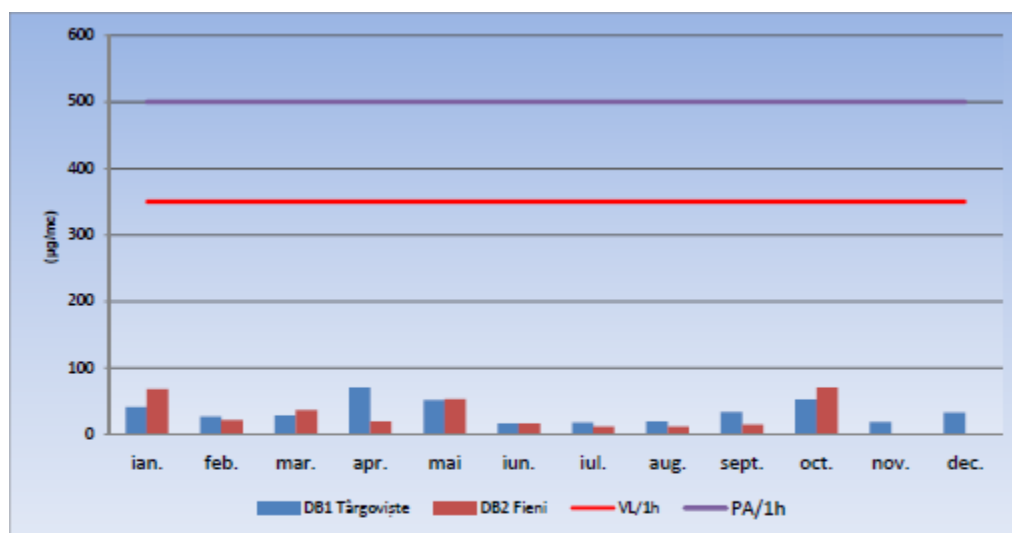
Grafic I.1.1.1.-1 Evoluția valorilor maxime lunare/1h ale indicatorului SO 2 , comparativ cu VL/1h și PA/1h pentru protecția sănătății umane
